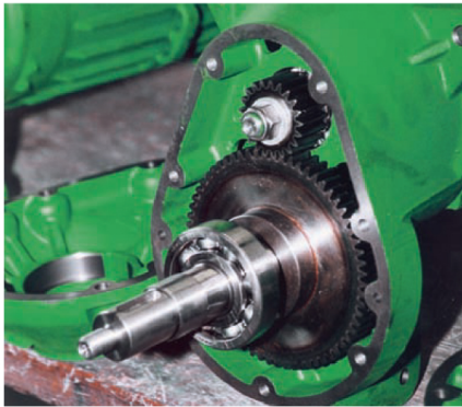
Stirnradgetriebe GTWS 740/1040
